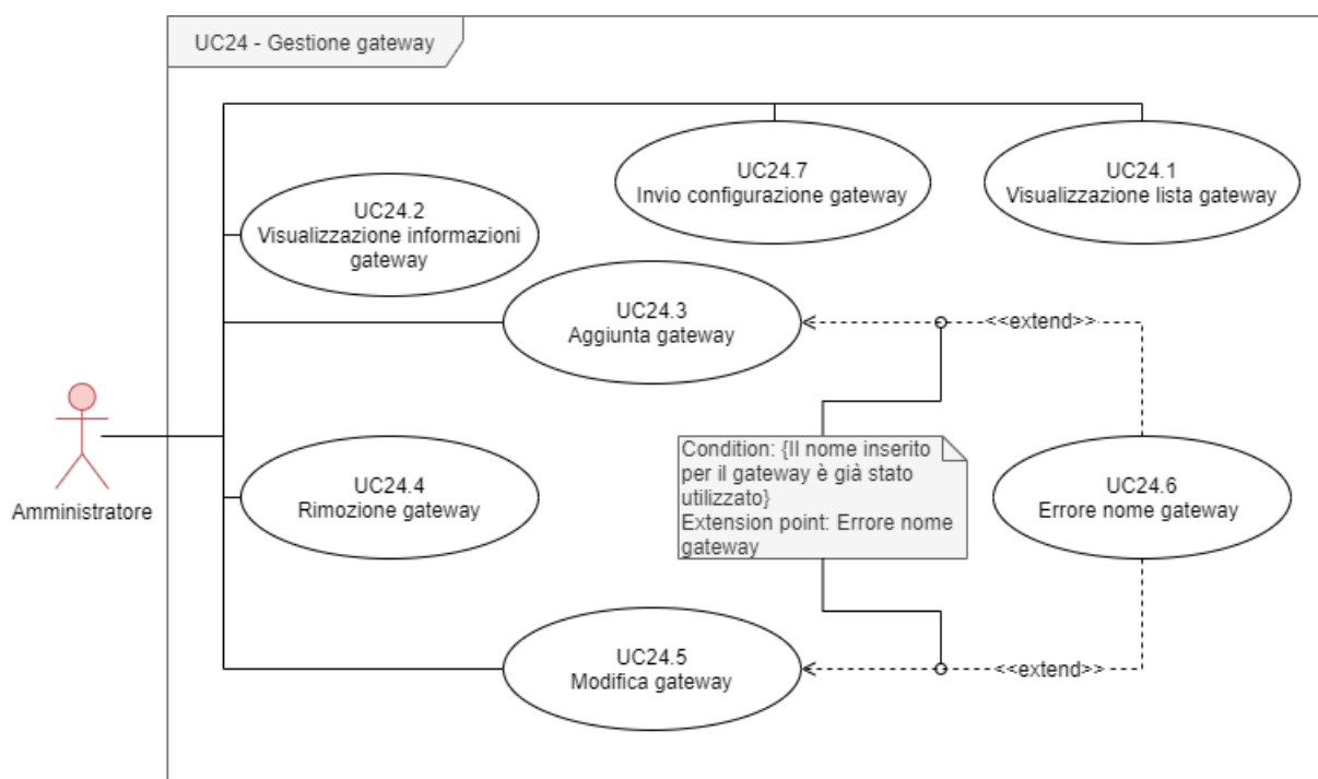
Figura 14: Diagramma che riassume la gestione dei gateway da parte dell'amministratore del sistema.
